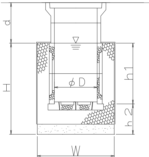
【標準構造図】EMC
