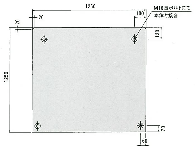
妻壁平面図
