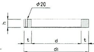
A-A 断面図
