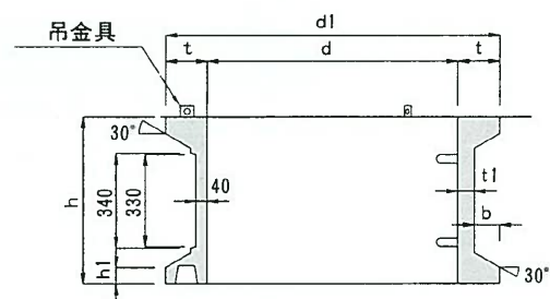
A-A 断面図
