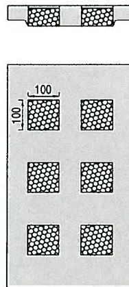
車道用
