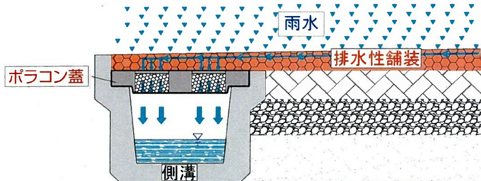
歩道用
