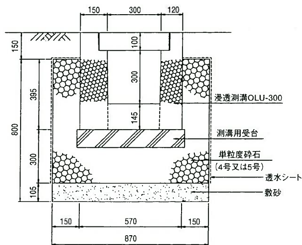
標準構造図
