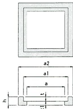
◆縁塊
