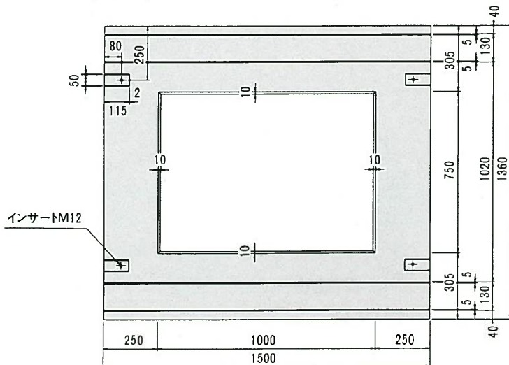
底板平面図
