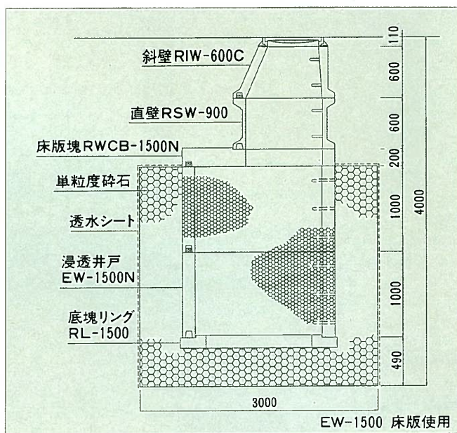
側面図
