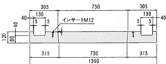
底板断面図
