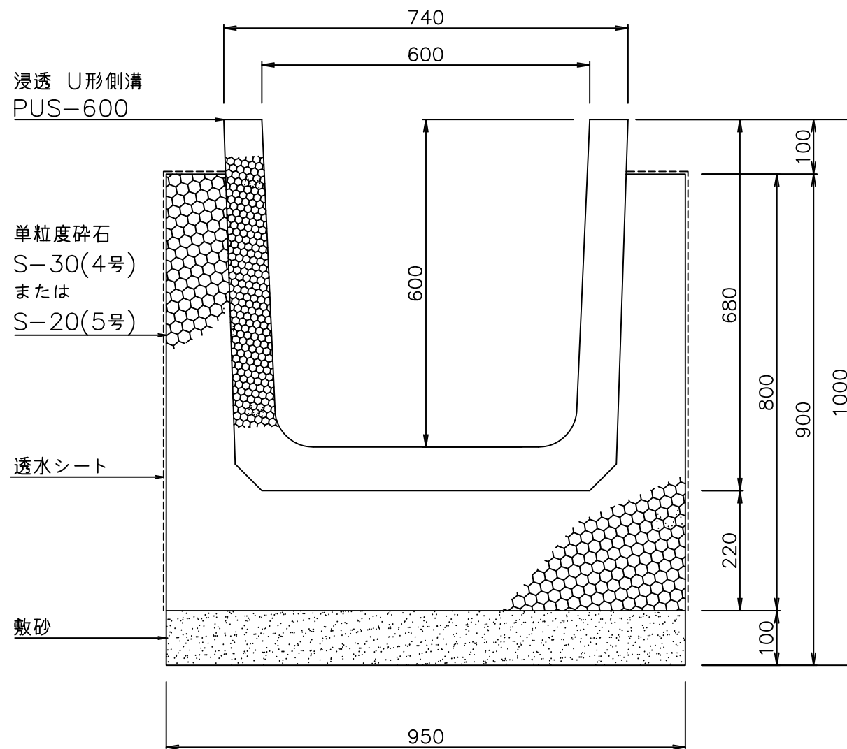
断面図
