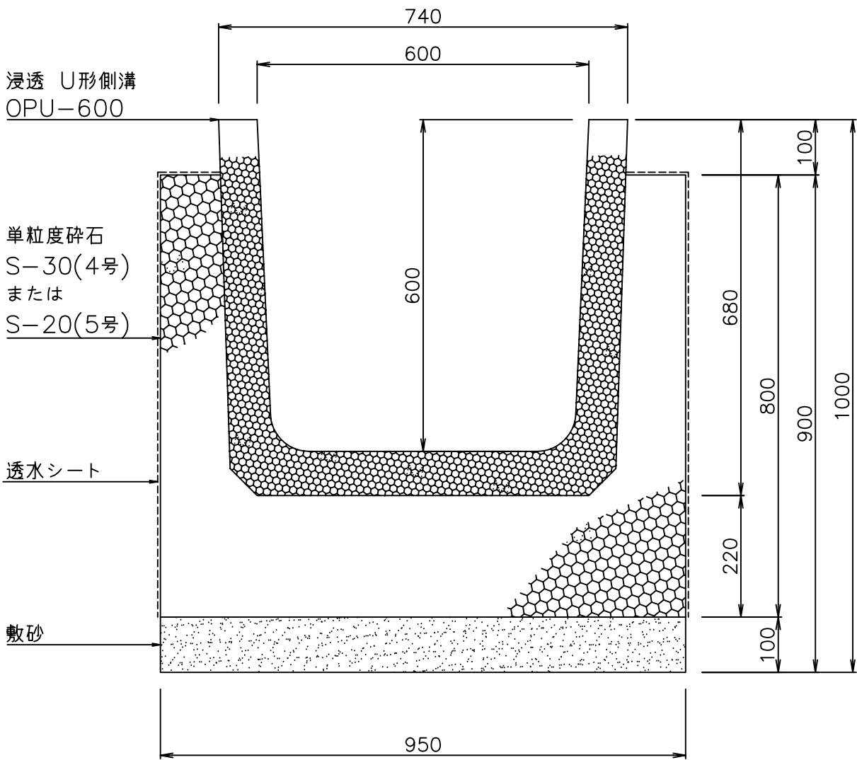
断面図
