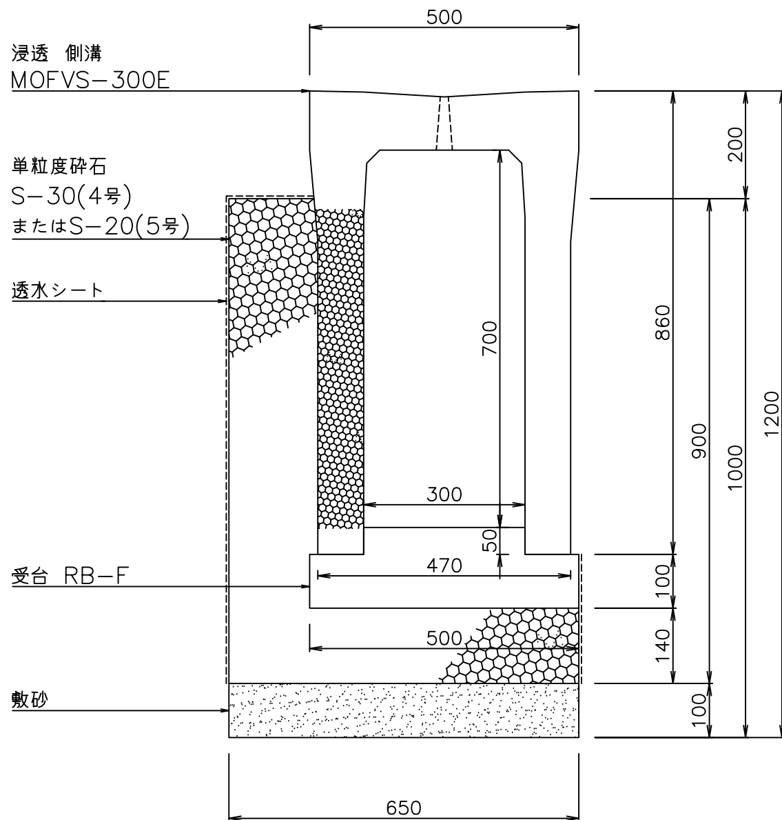
断面図
