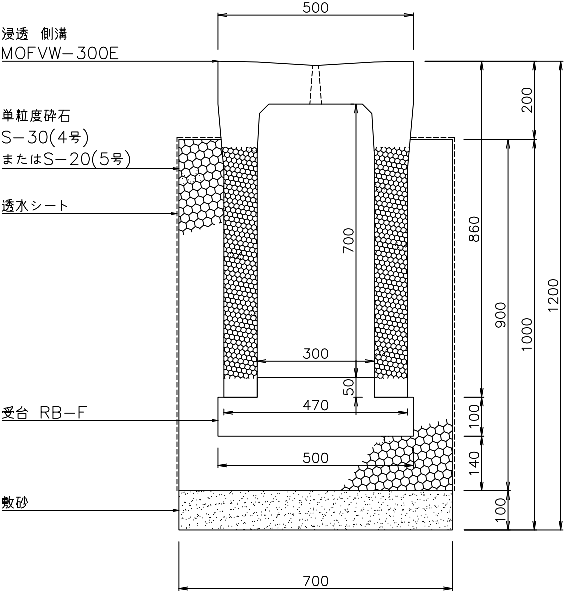
断面図
