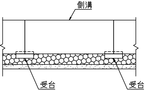
側面図
