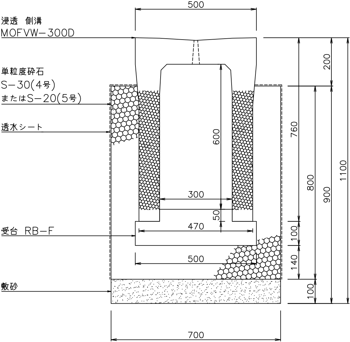
断面図
