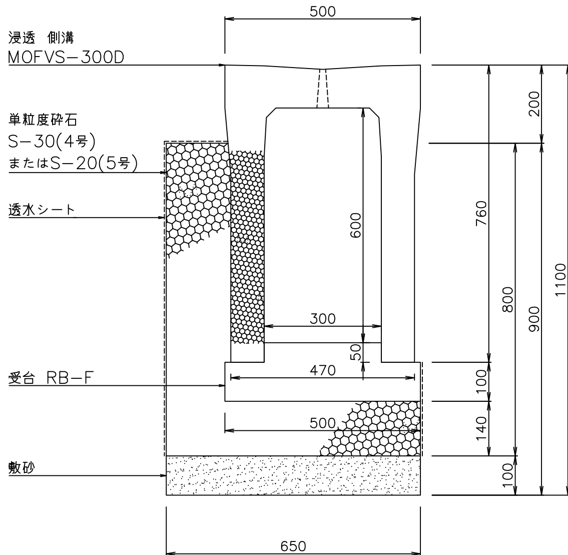
断面図
