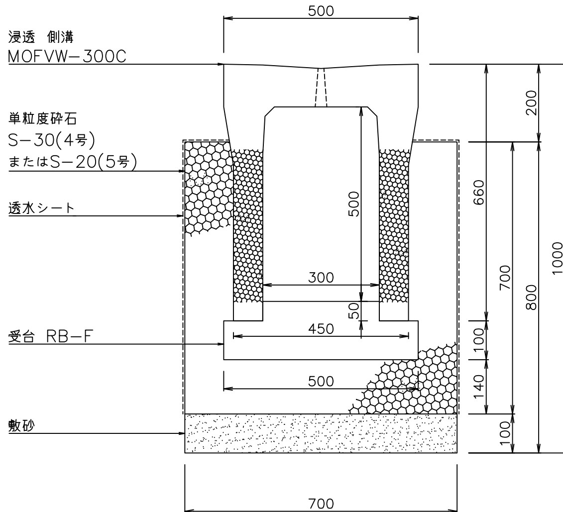
断面図
