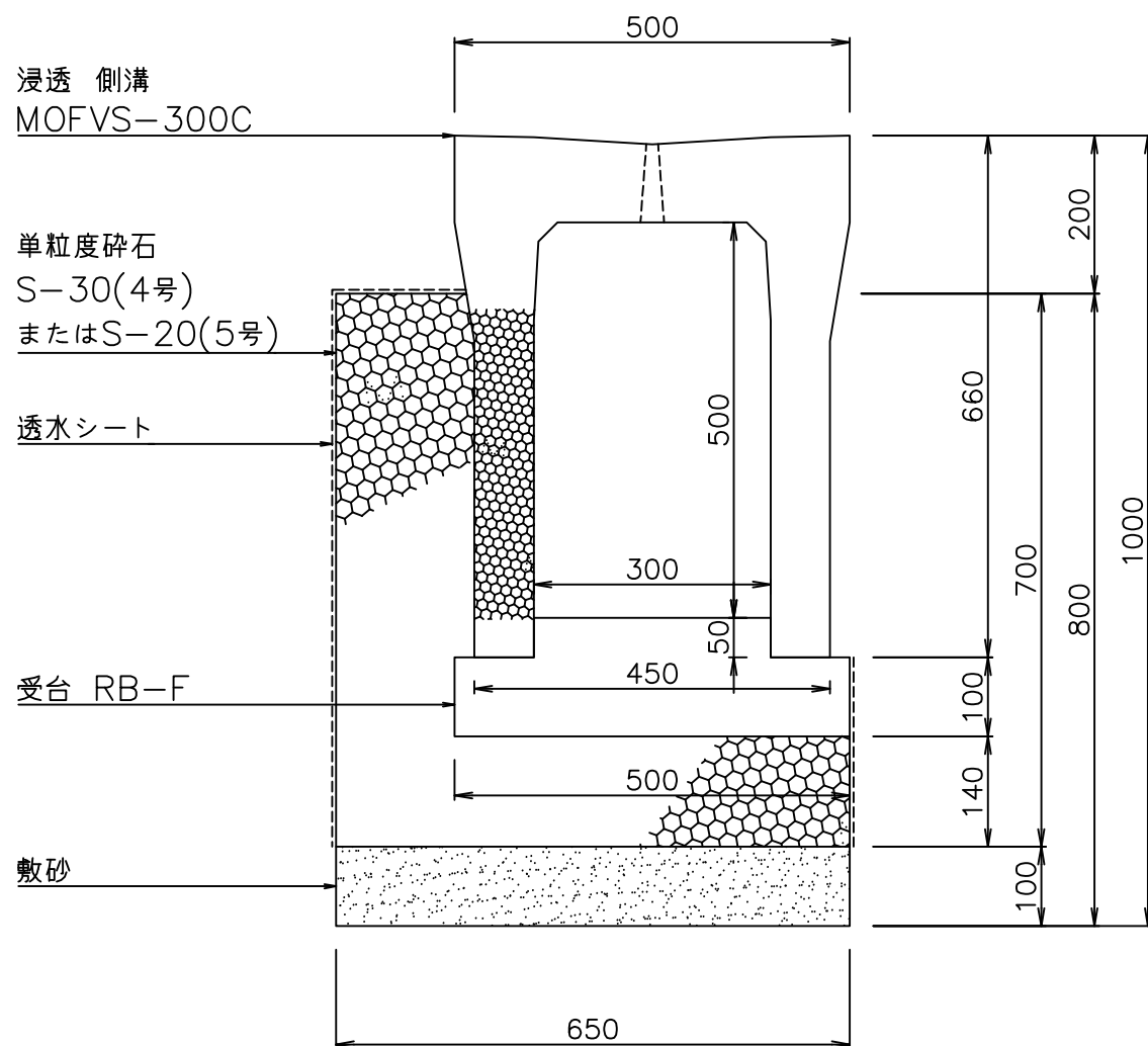
断面図
