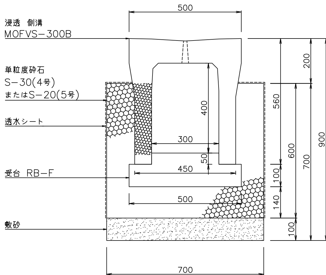
断面図
