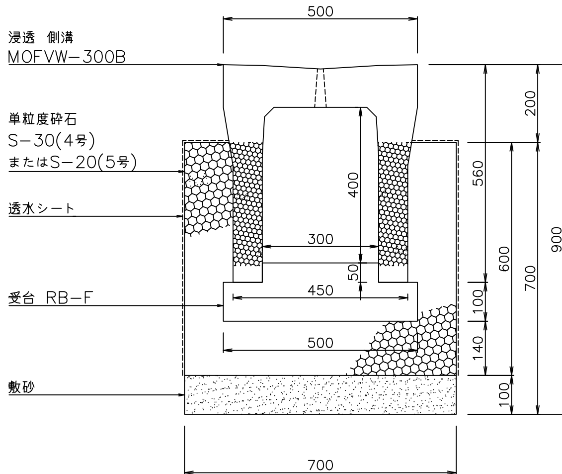
断面図
