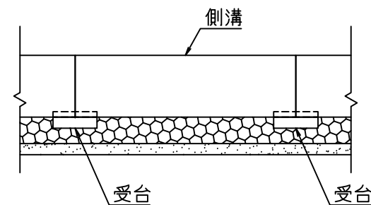
側面図
