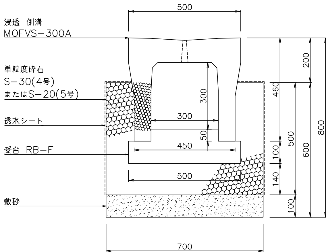
断面図
