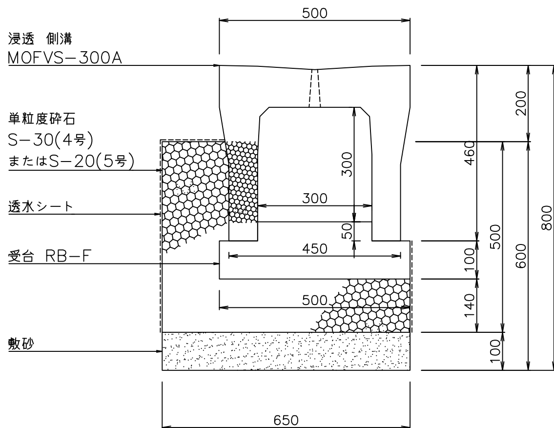
断面図
