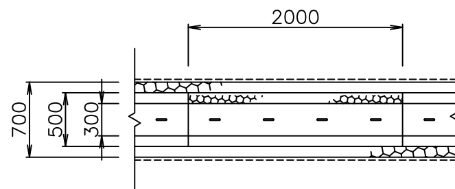
平面図
