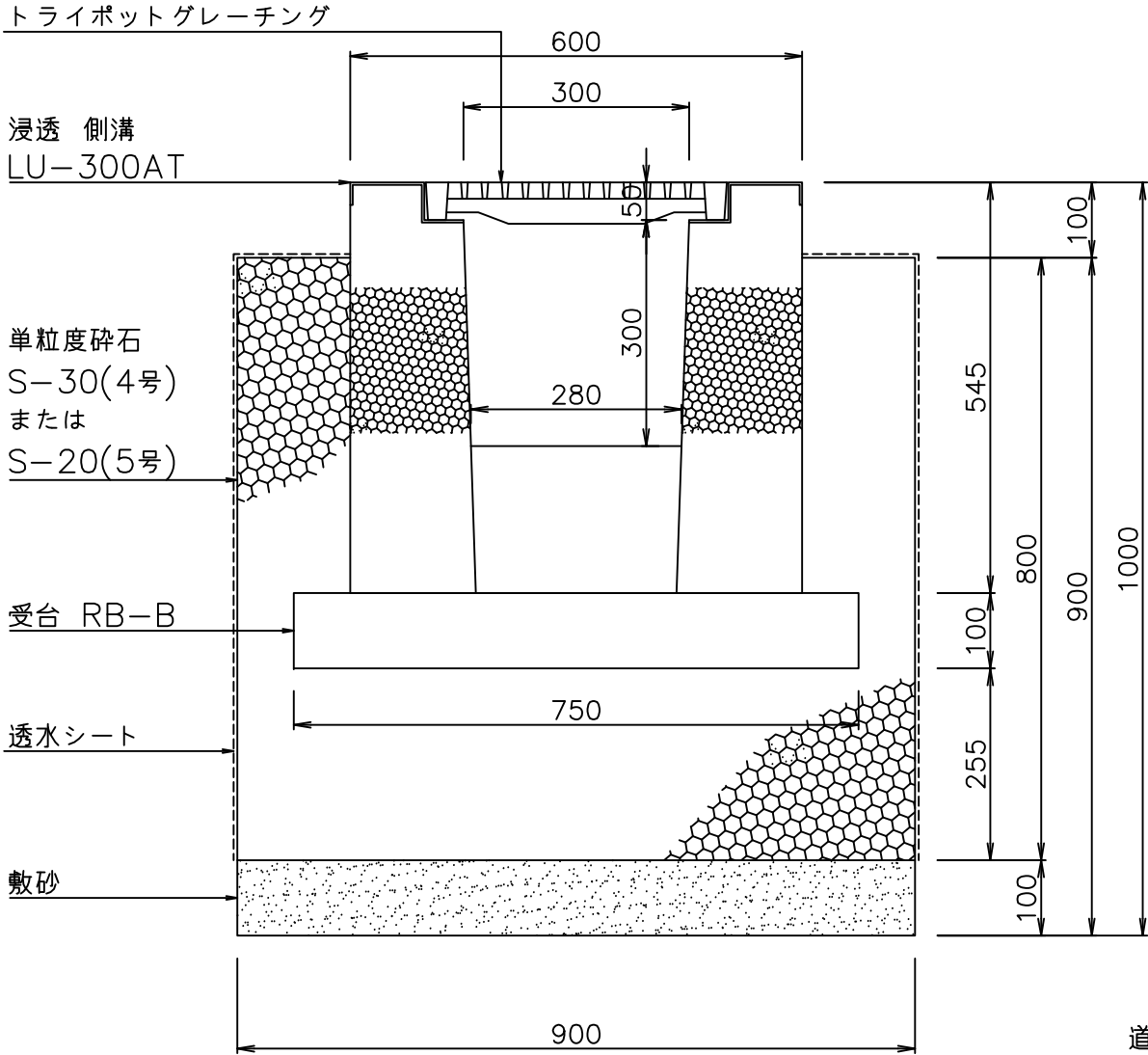
断面図
