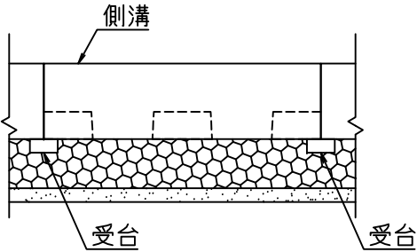
側面図
