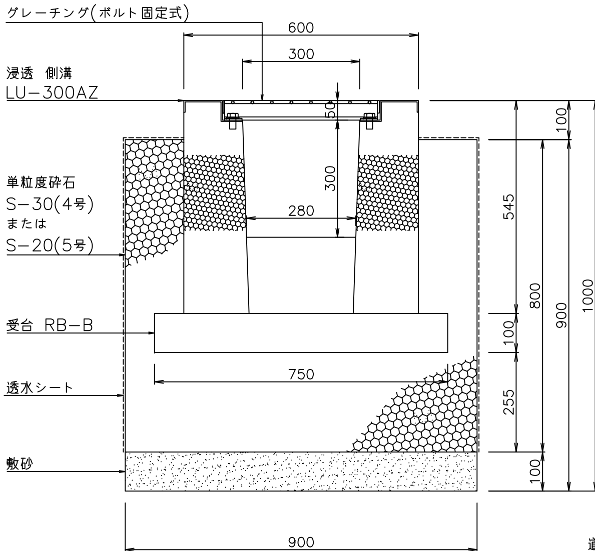
断面図
