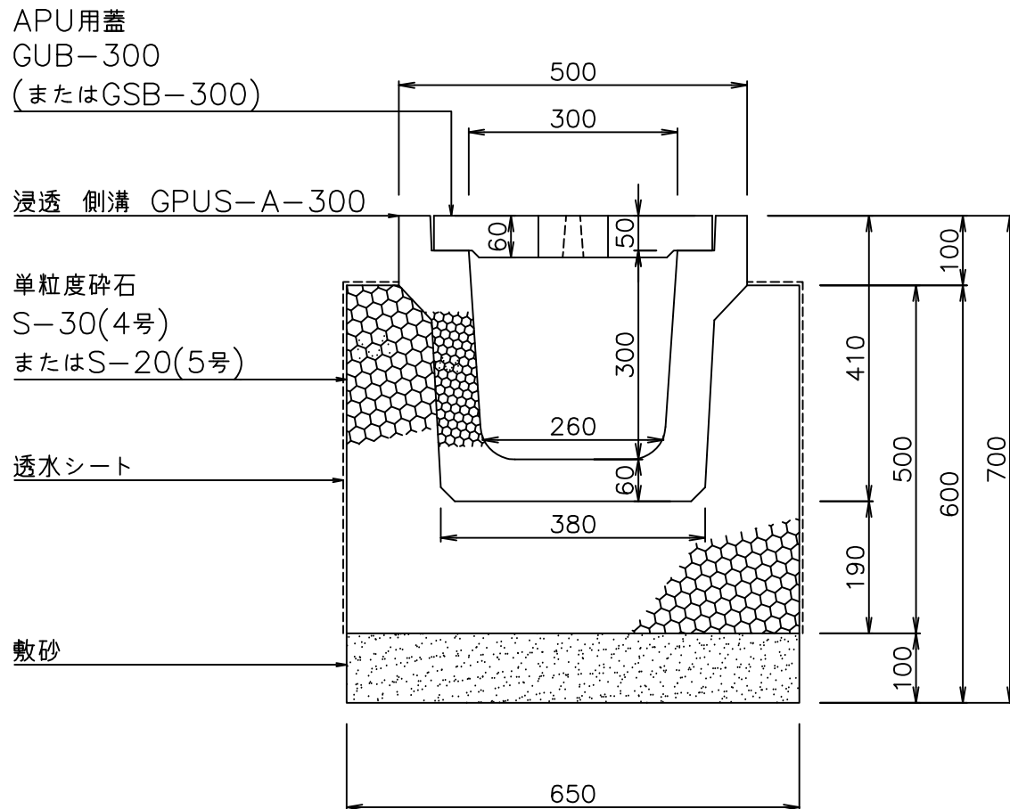
断面図
