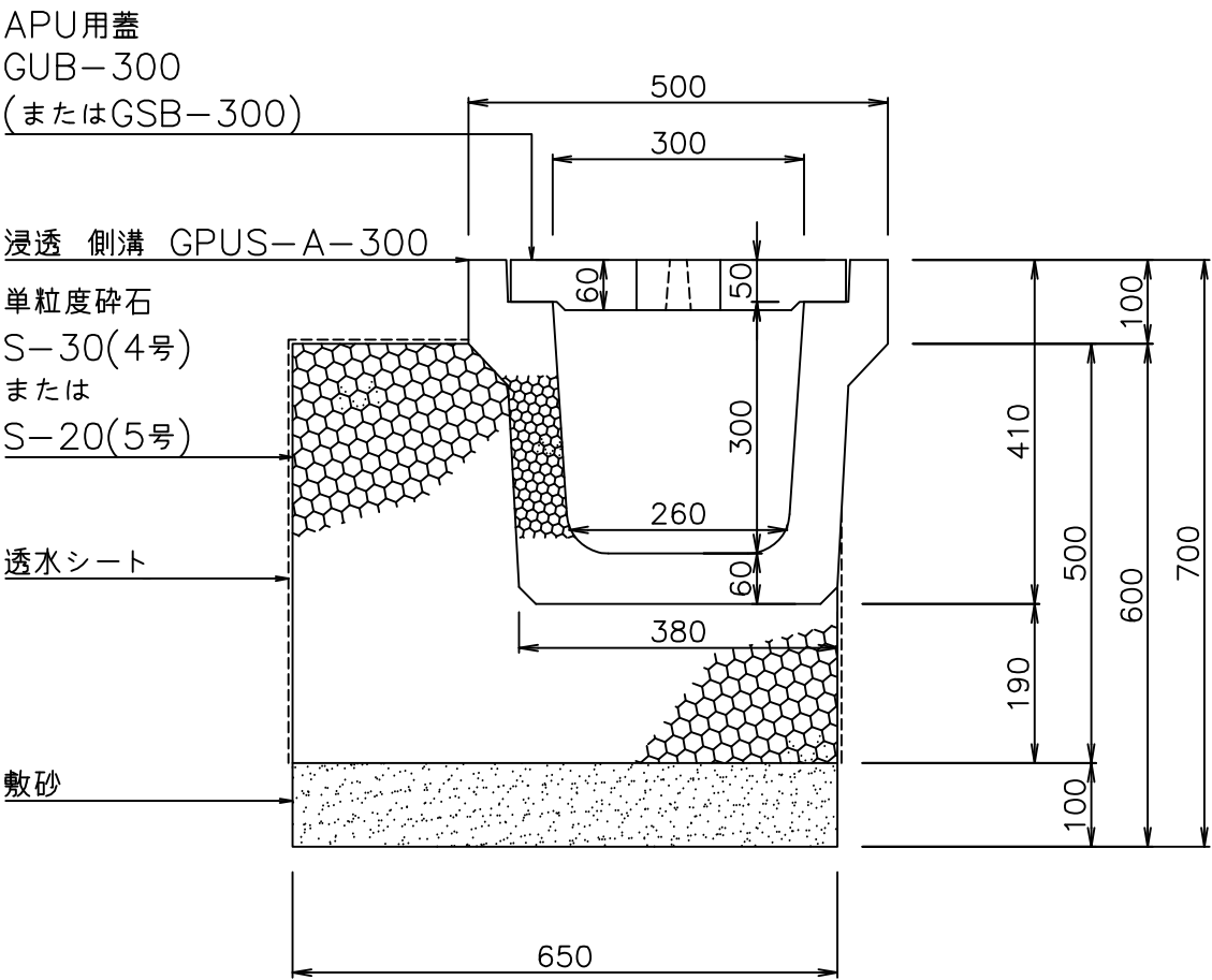
断面図
