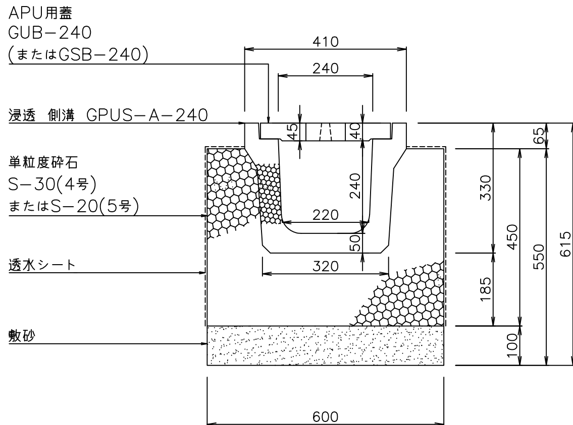
断面図
