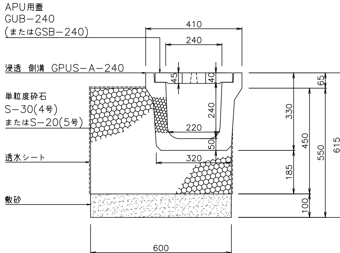
断面図
