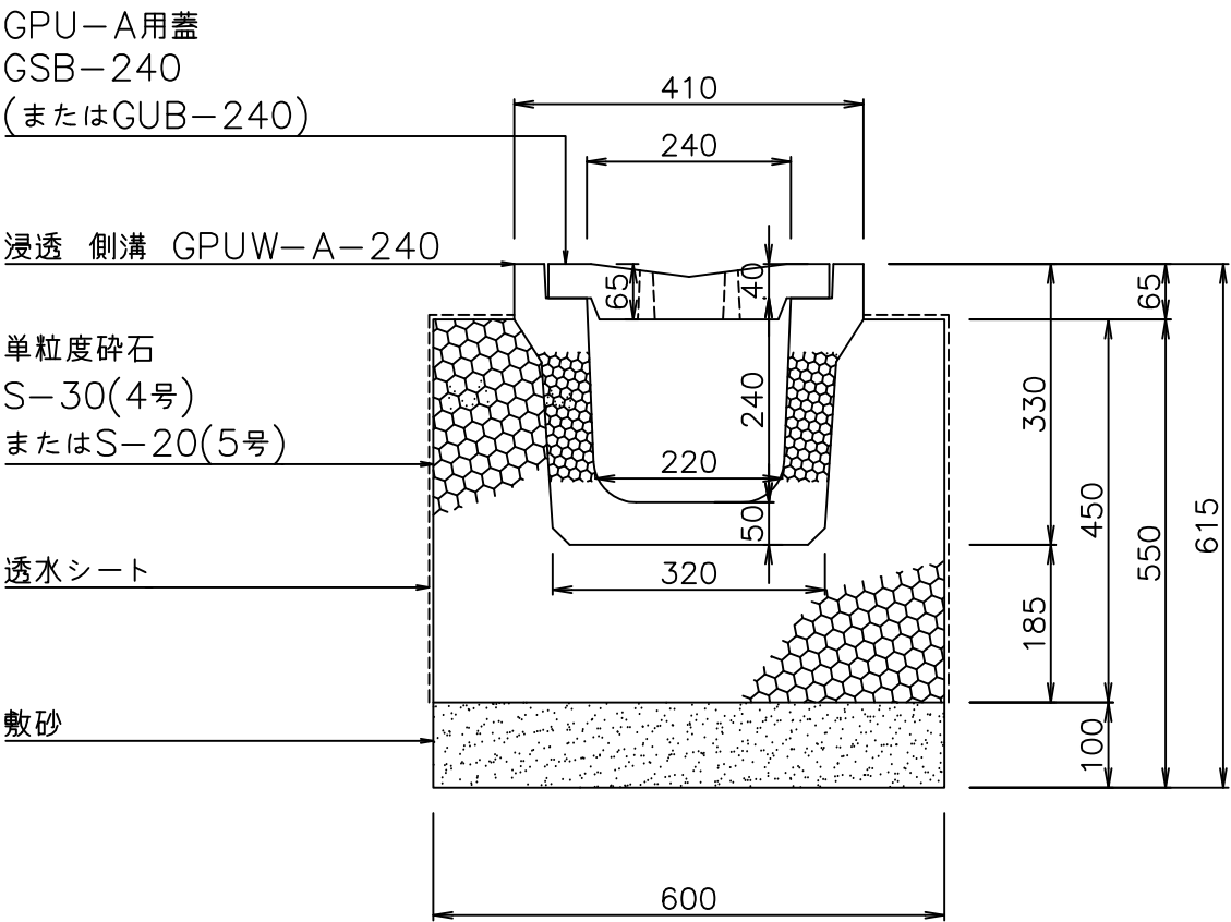
断面図
