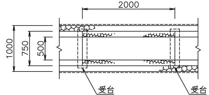
平面図
