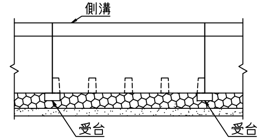
側面図
