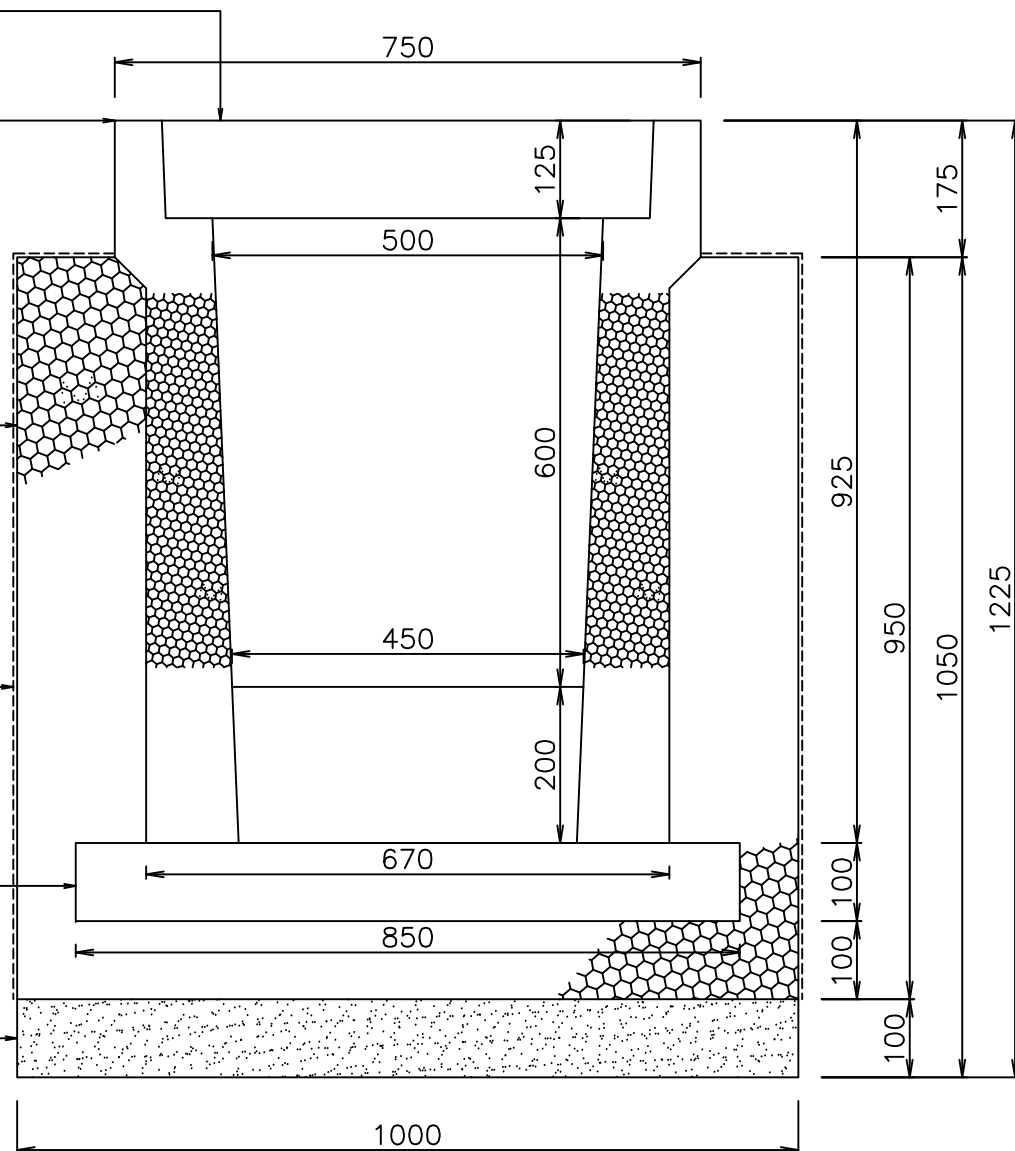
断面図
