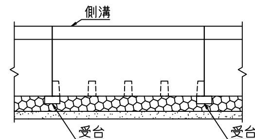
側面図
