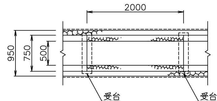
平面图
