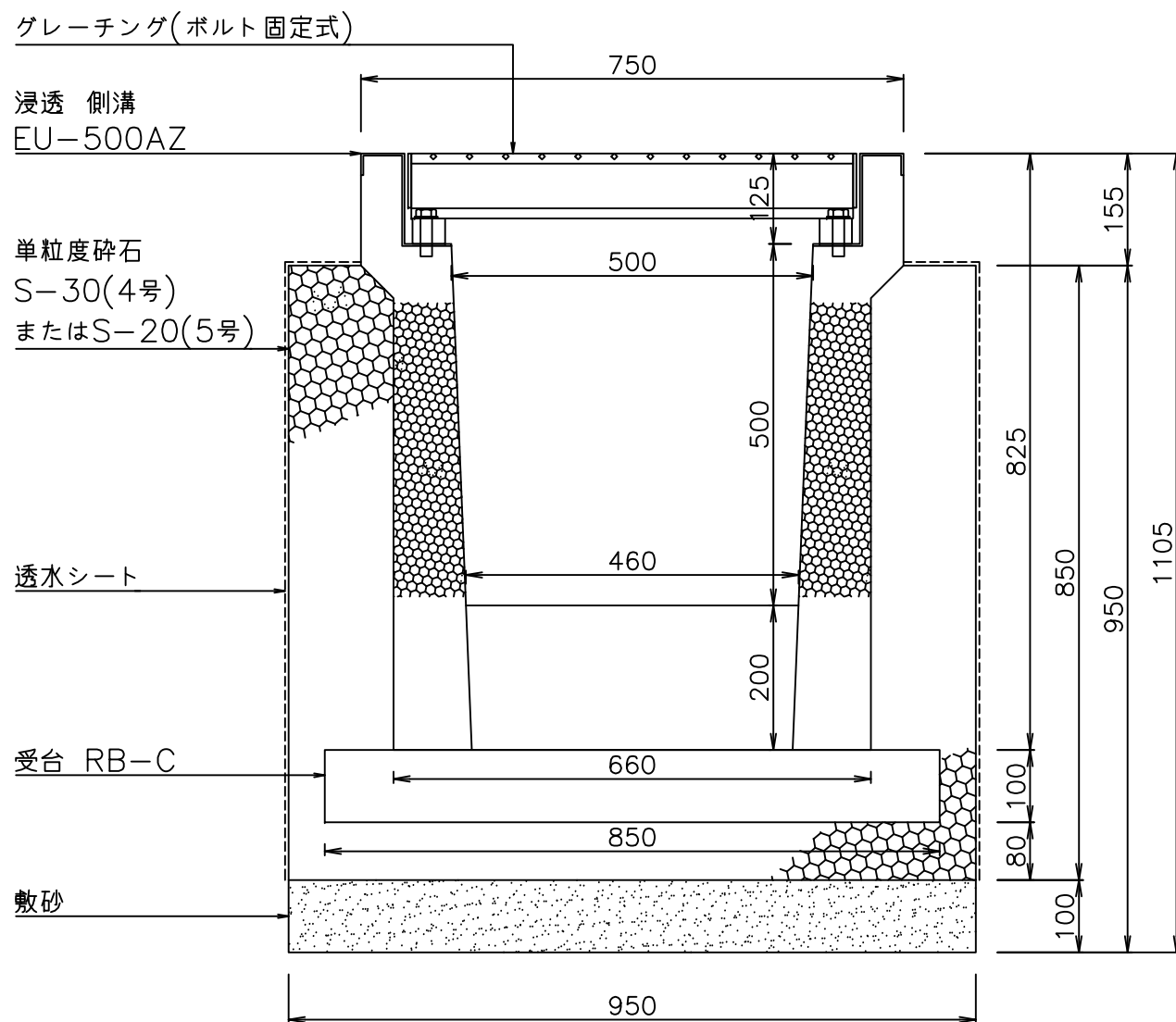
断面図
