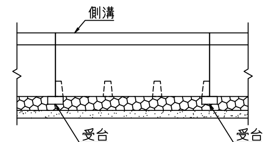
側面図
