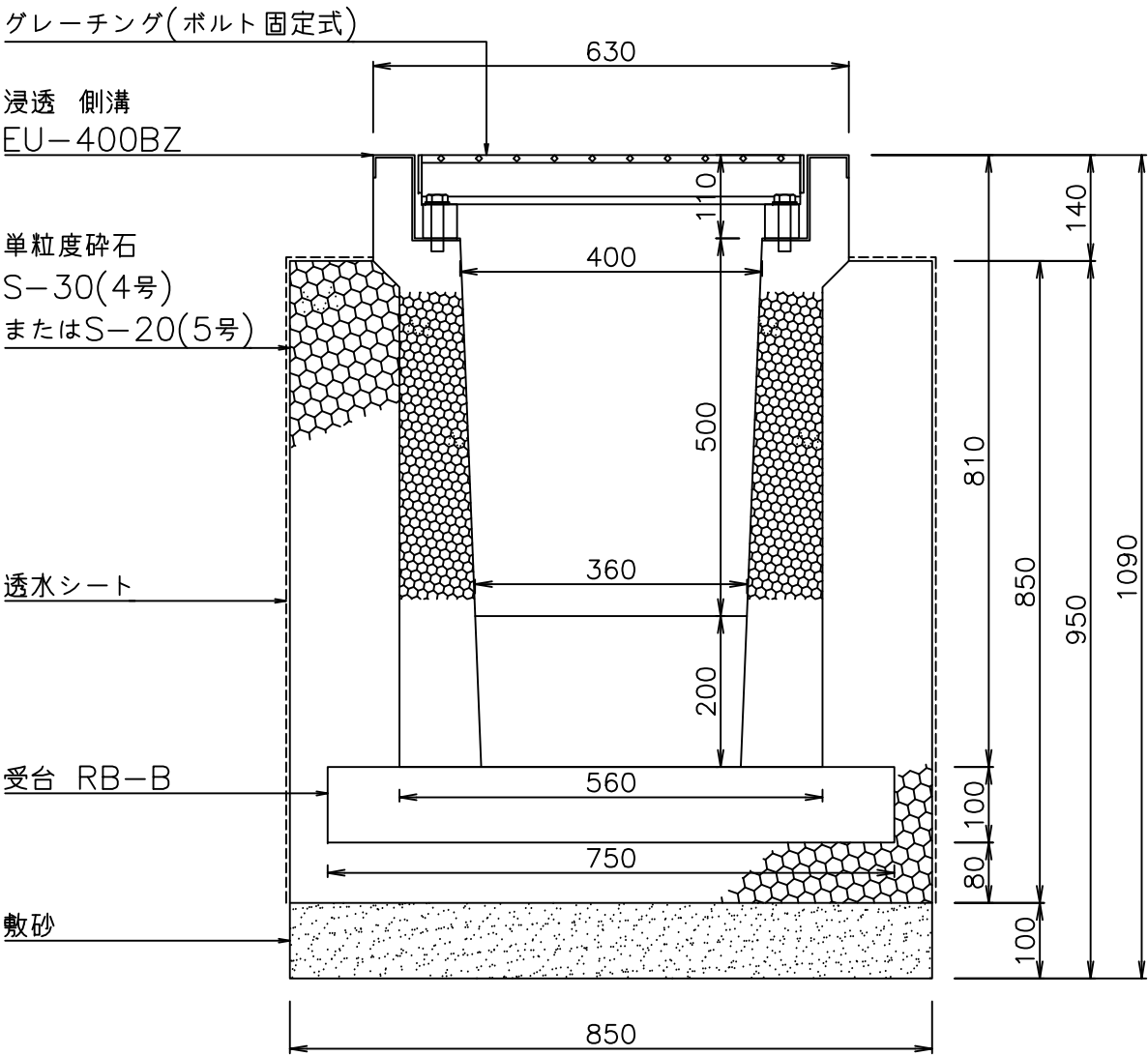
断面図
