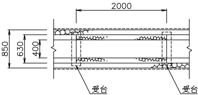
平面図
