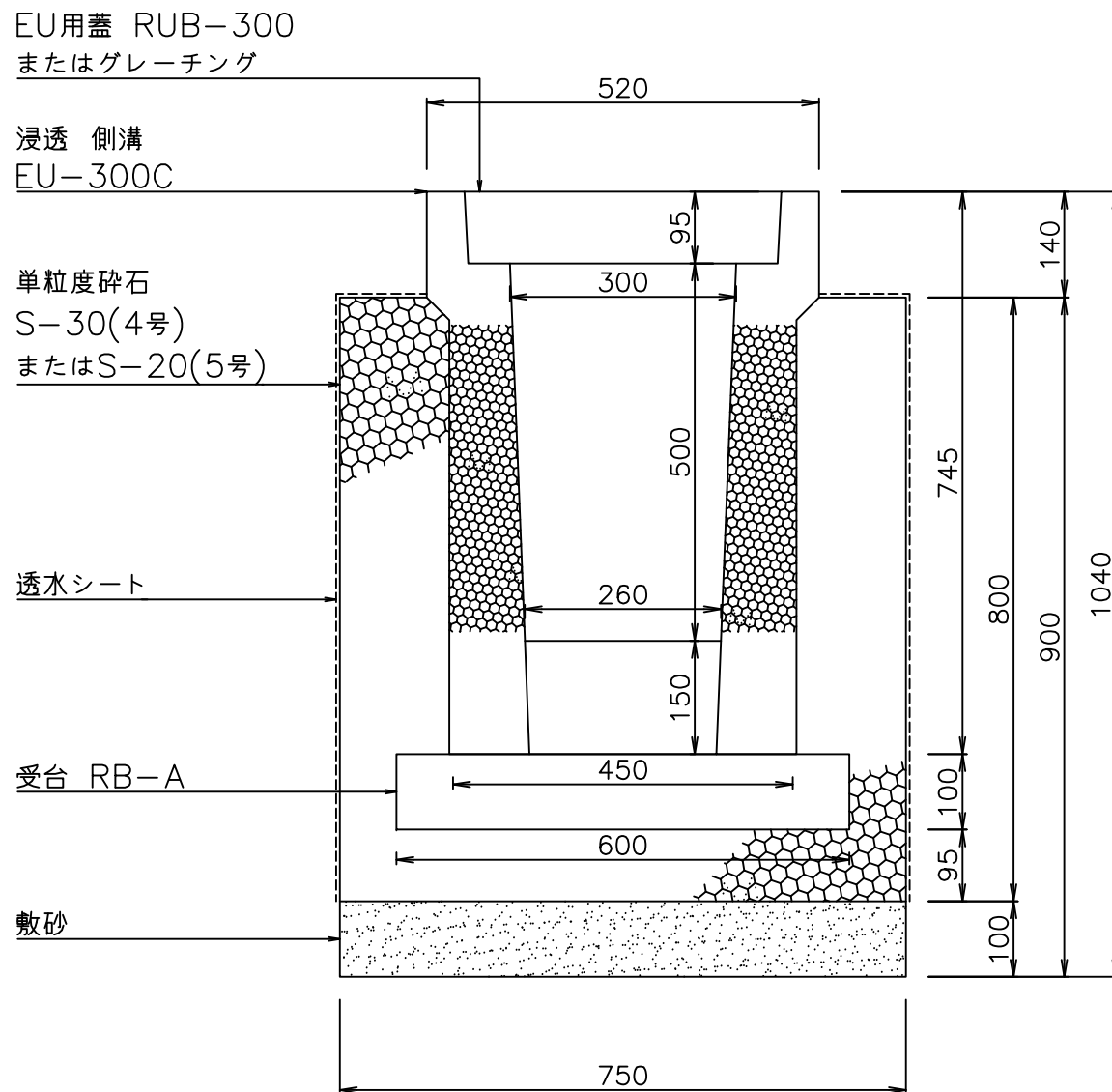
断面図
