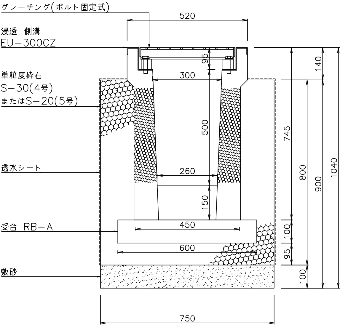
断面図
