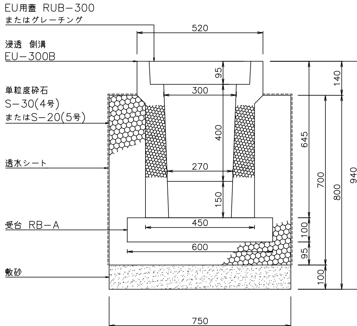
断面図
