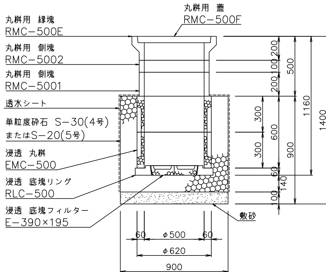
断面図
