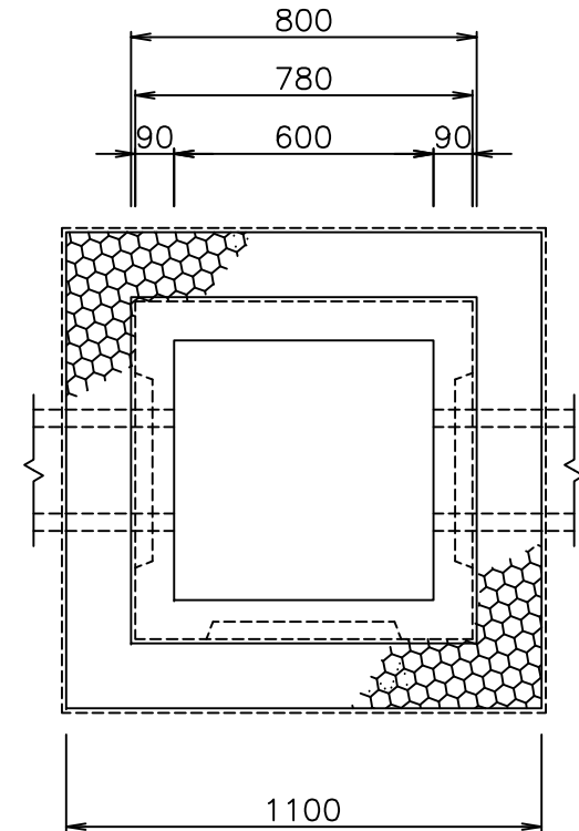
平面図
