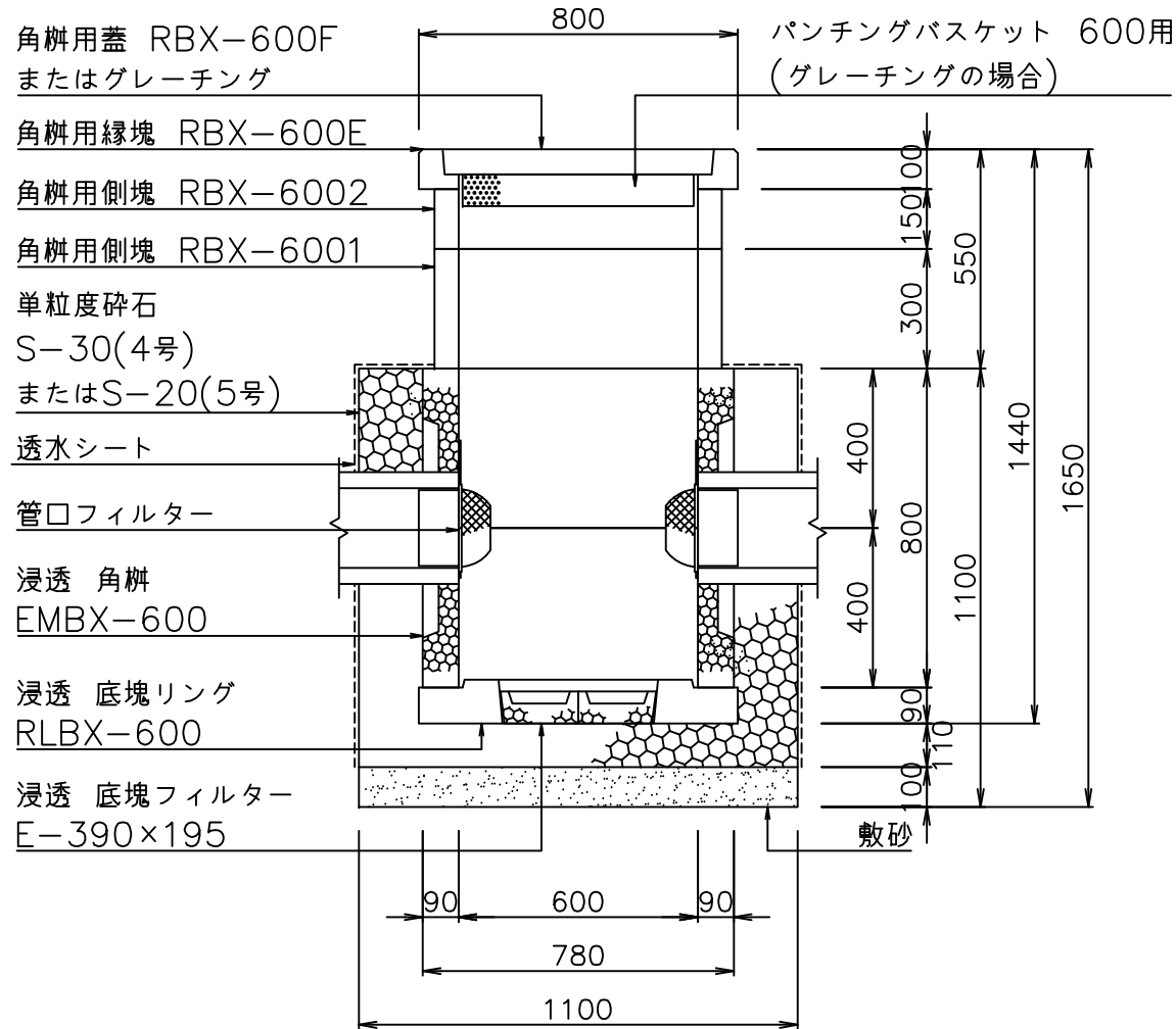
断面図
