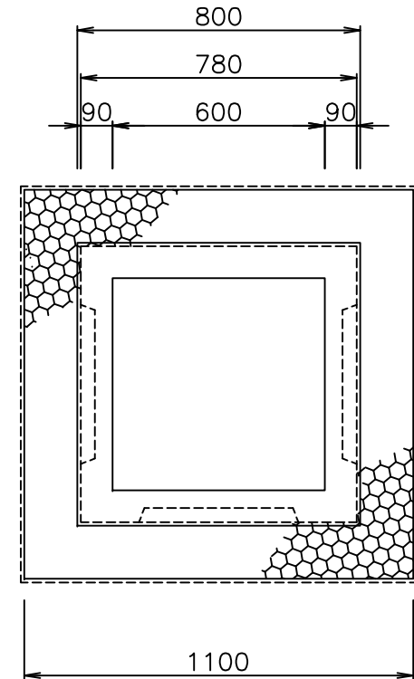
平面図
