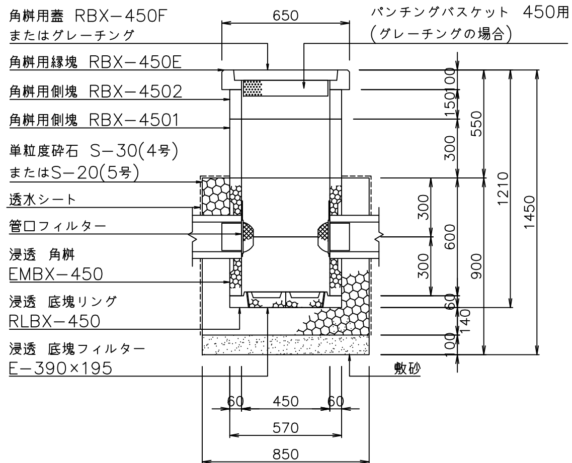
断面図
