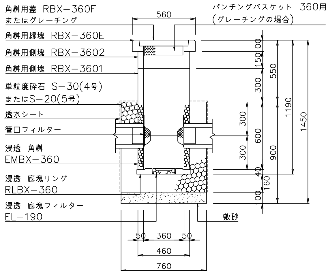
断面図
