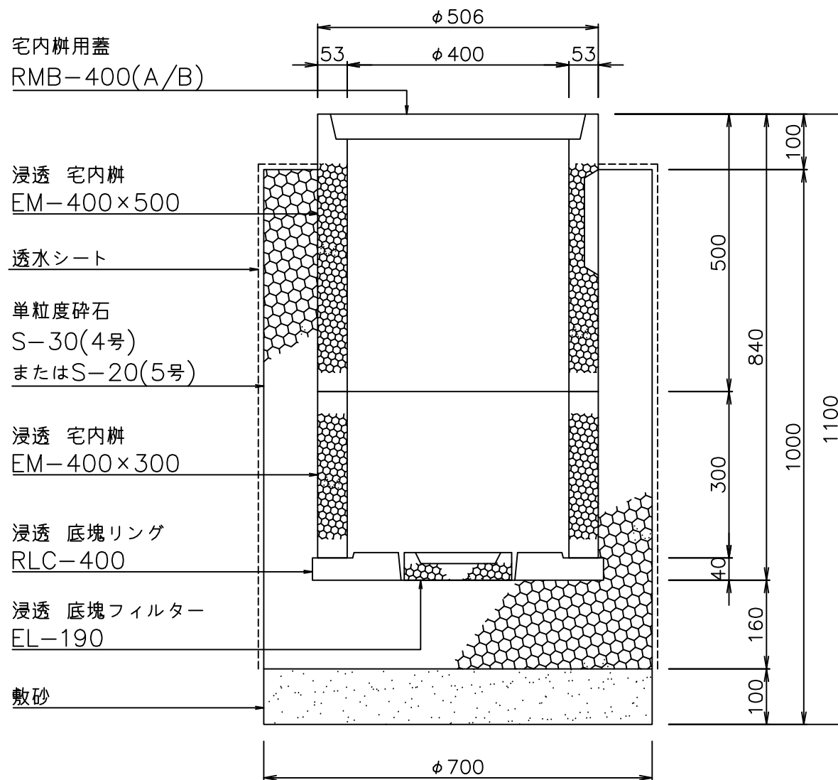
断面図
