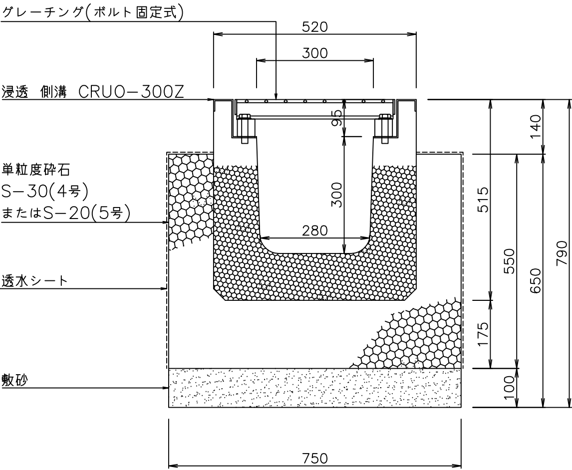
断面図
