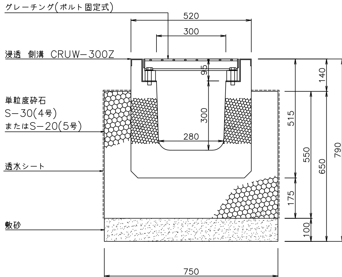
断面図
