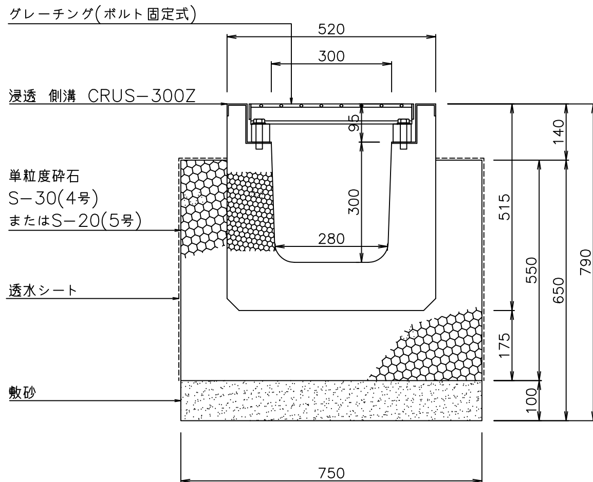
断面図
