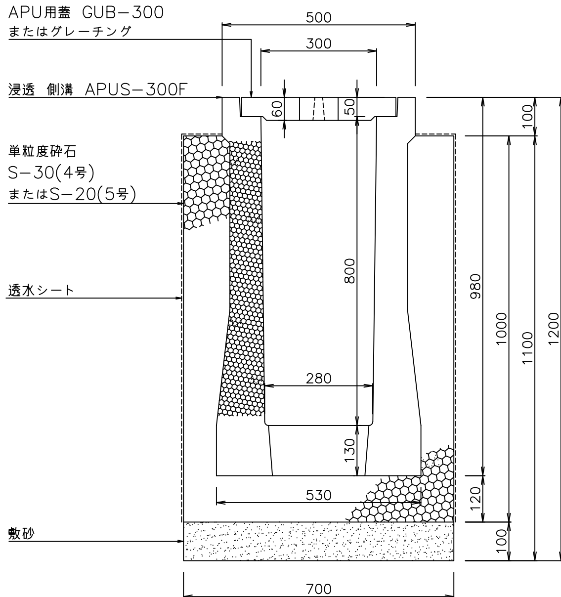
断面図
