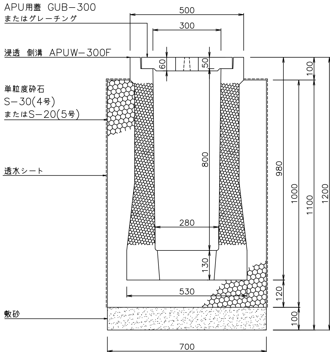
断面図
