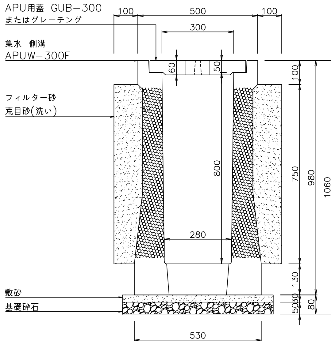
断面図
