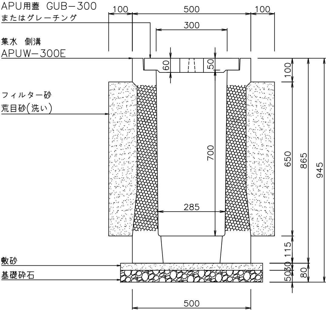
断面図
