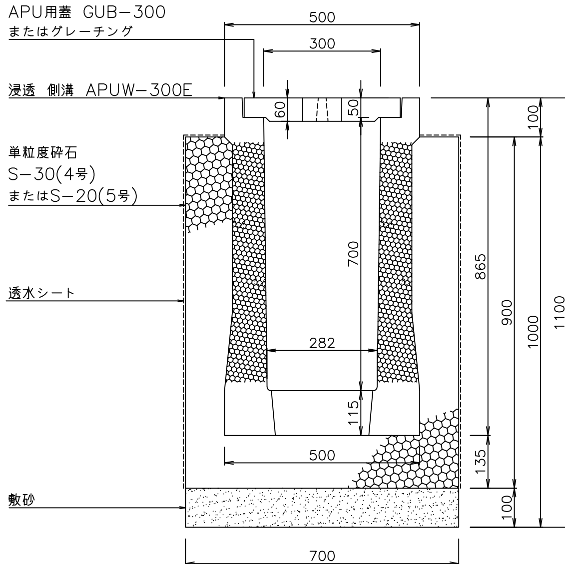
断面図
