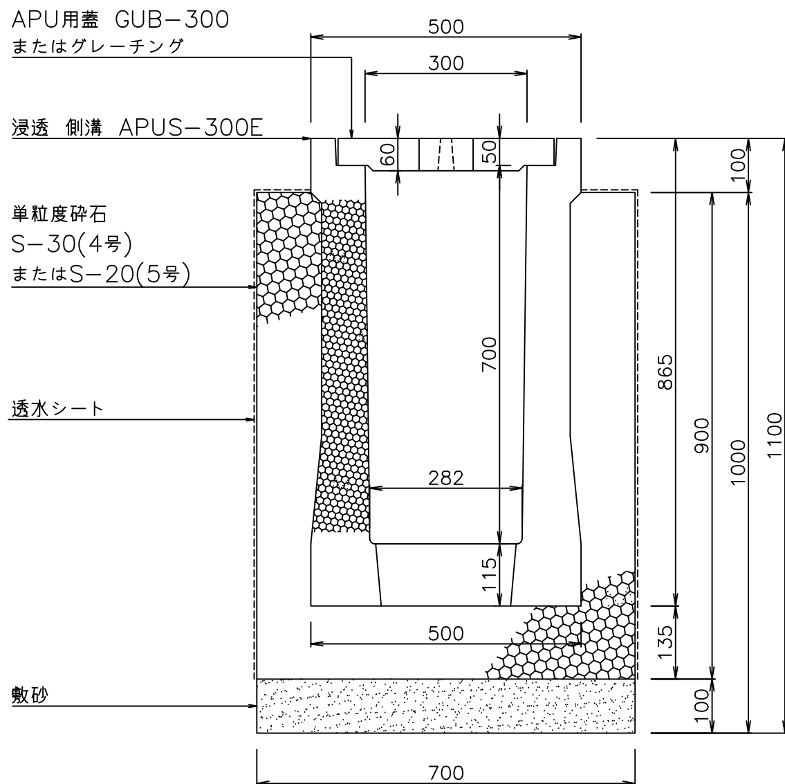
断面図
