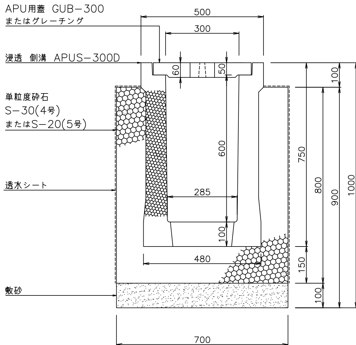
断面図
