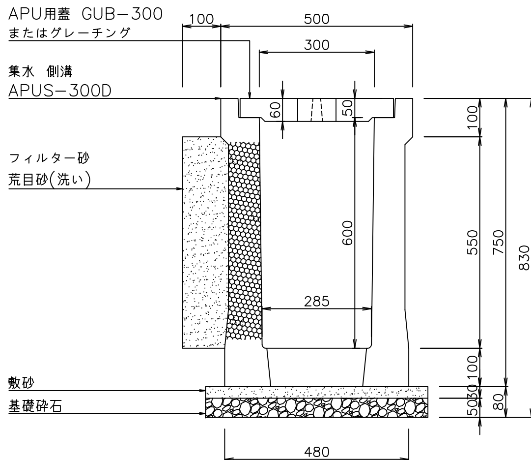
断面図
