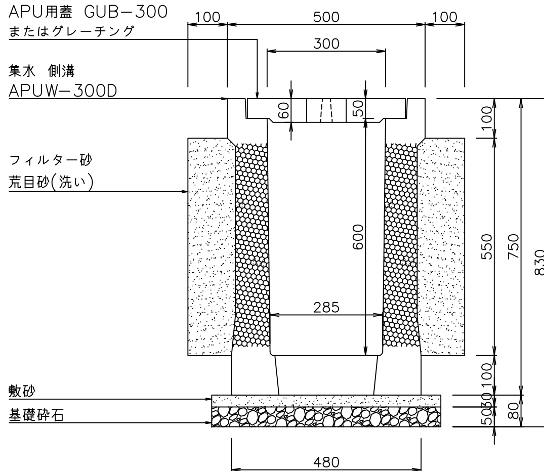
断面図
