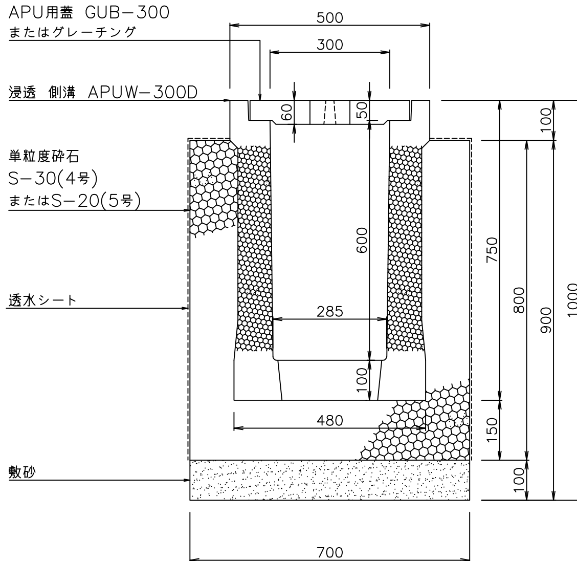
断面図
