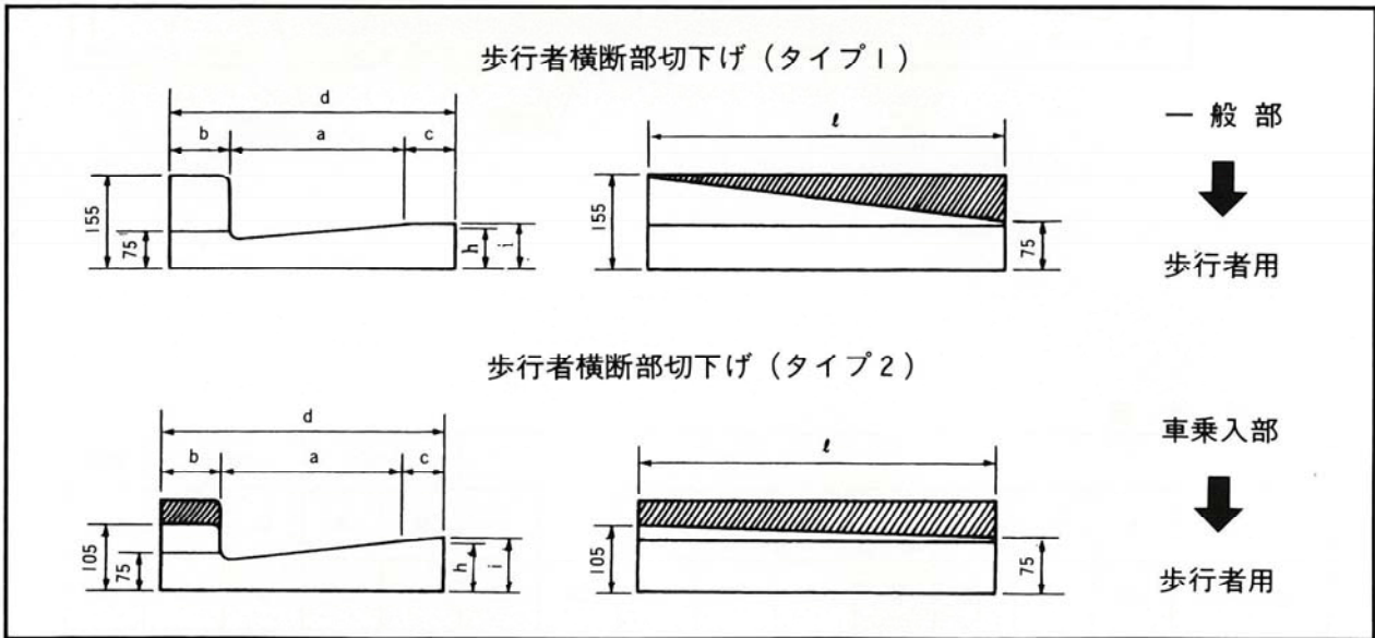
鉄筋コンクリートL形（歩行者横断用）
