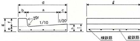
鉄筋コンクリートL形
