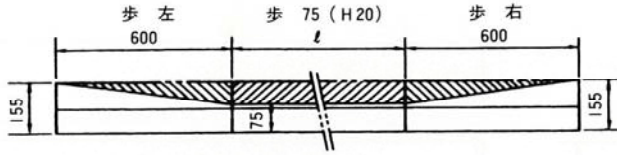
歩行者横断部左右（タイプ1）
