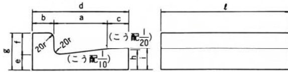
コンクリートL形
