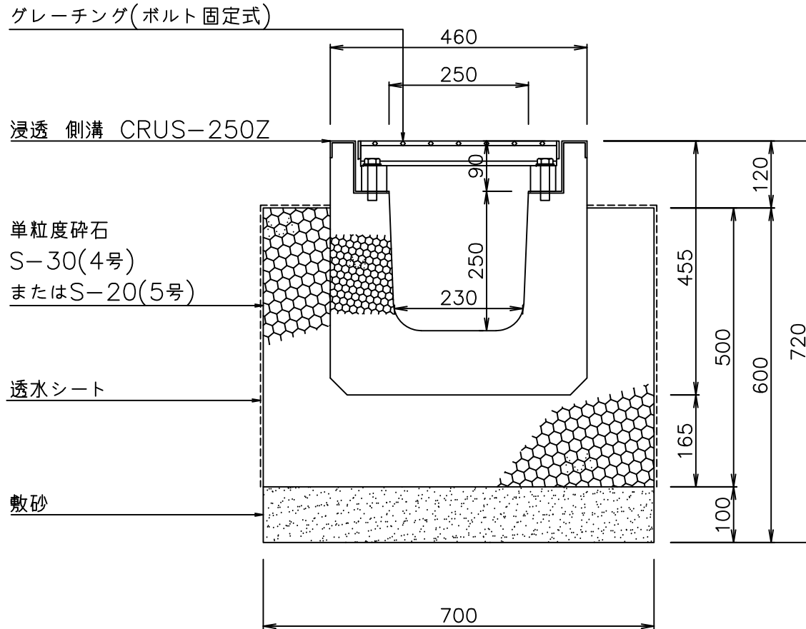
断面図
