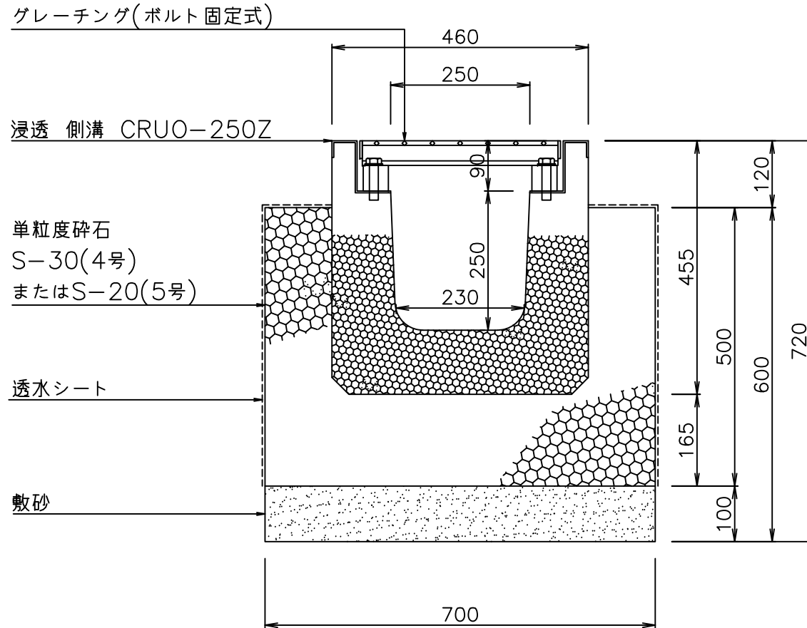
断面図
