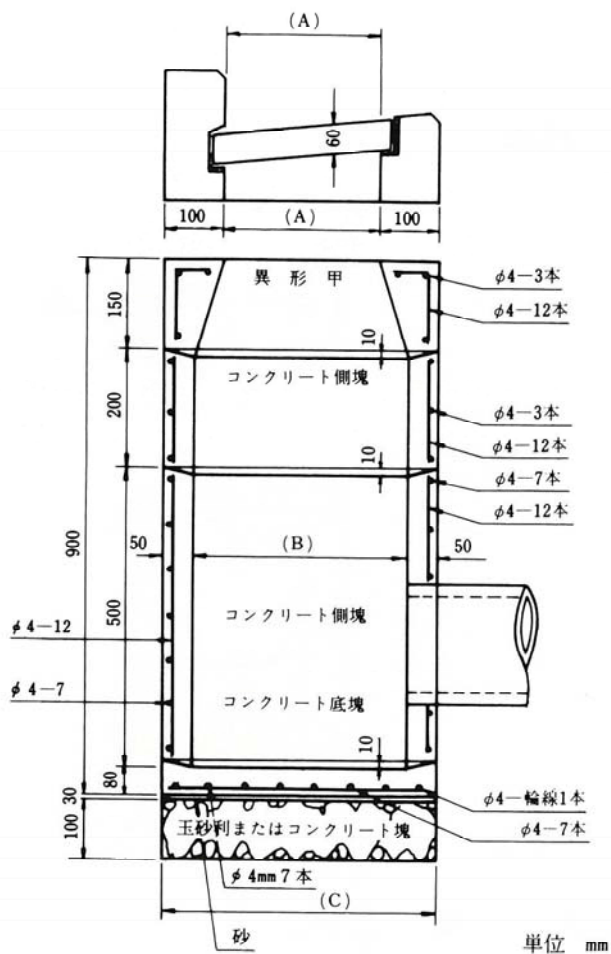
L形集水樹躯体
