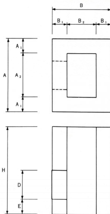
L形集水樹躯体
