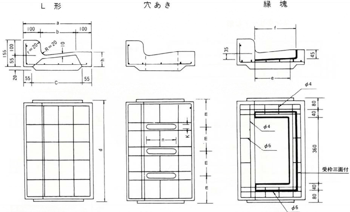
寸法表
